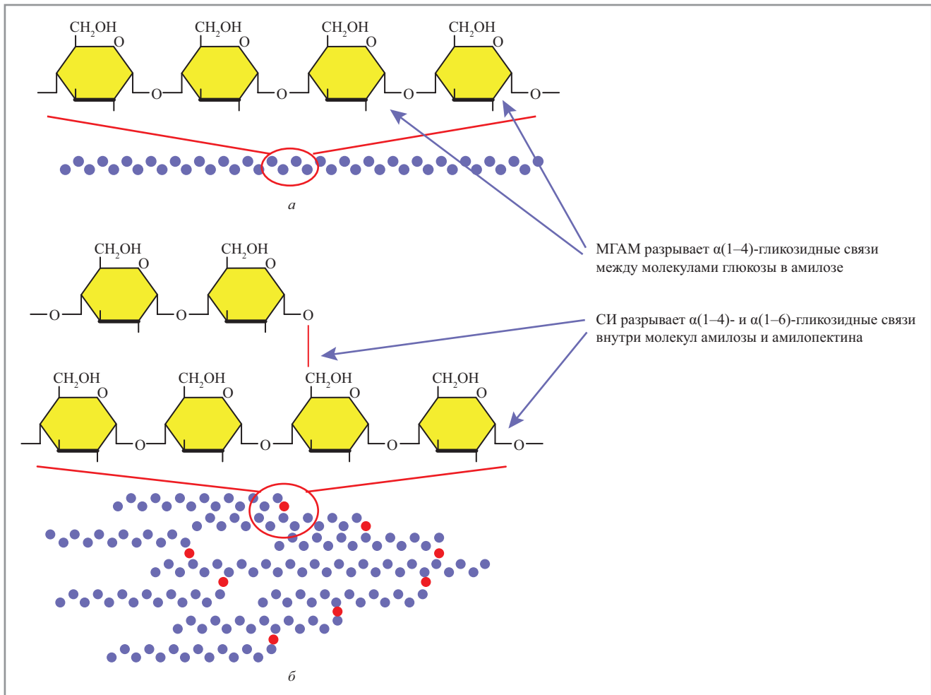
Рис. 2. Структура амилозы и амилопектина [7].
